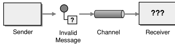
Invalid Message
